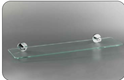
A4011BRM/C Repisa de metacrilato para complementos y amenities Dimensiones: 500 x 120 x 62 mm
