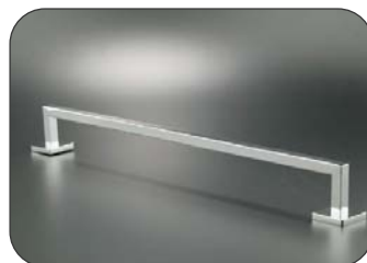
A2312BRB Toallero de barra recto de 60 cm Doble apoyo a pared de tubo cuadrado de 16 mm. Dimensiones: 634 x 75 x 50 mm
